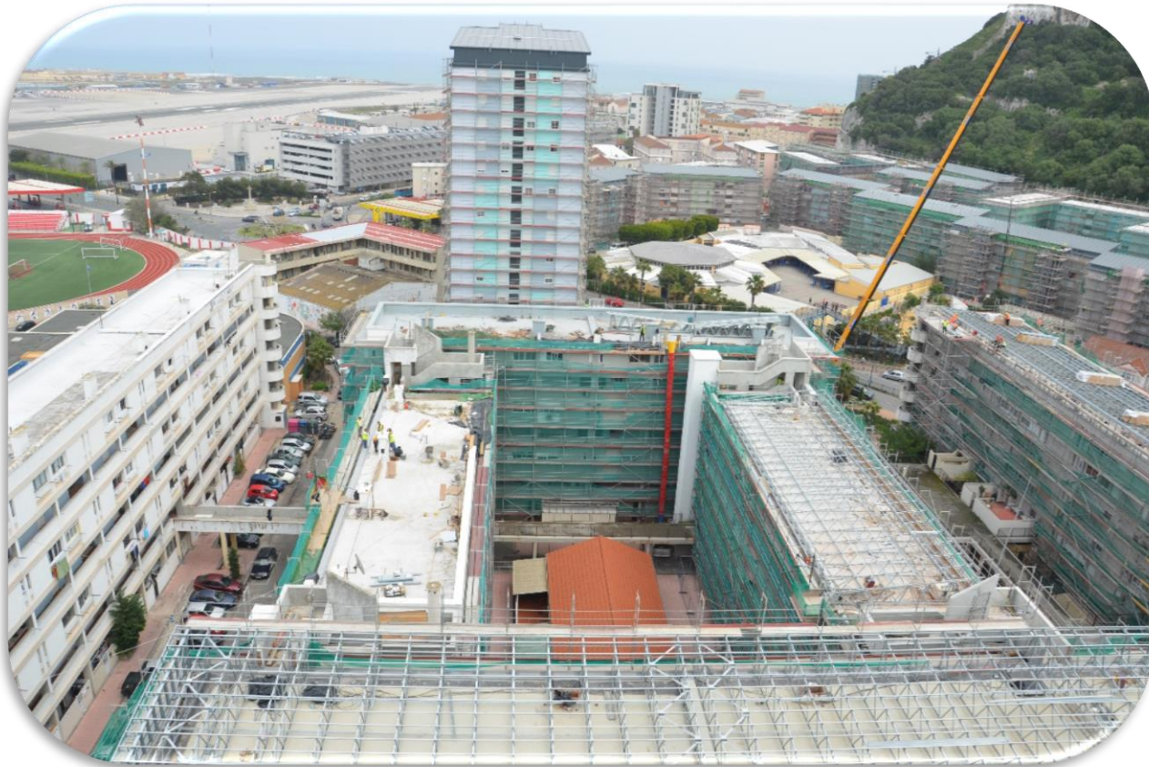
Rehabilitación integral de la barriada de la Laguna en la que se interviene 27 bloques
