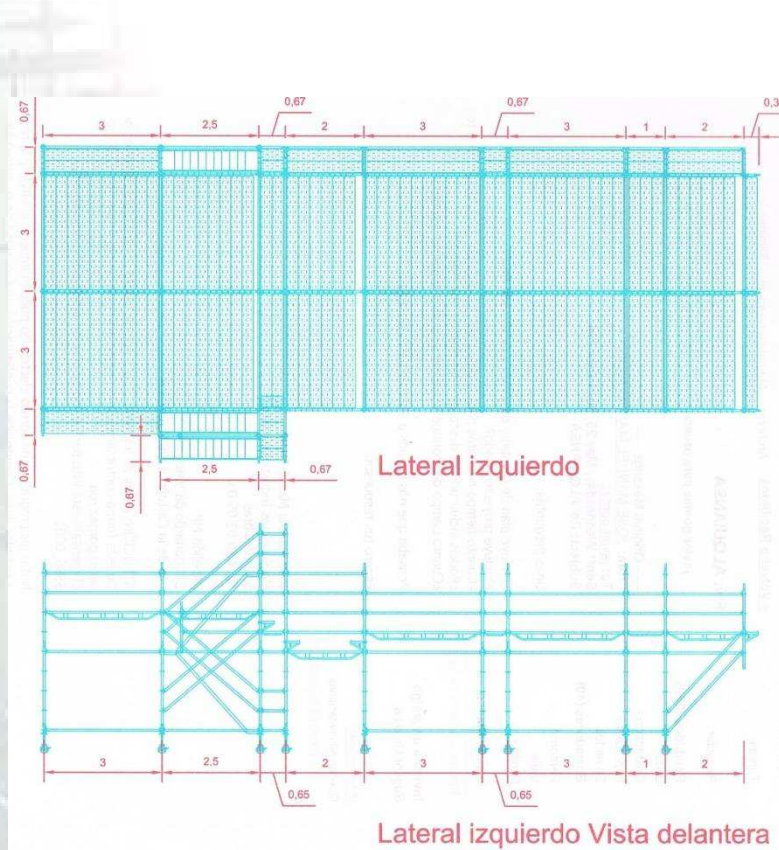
Planta y alzado de gradas para reparación de aviones
