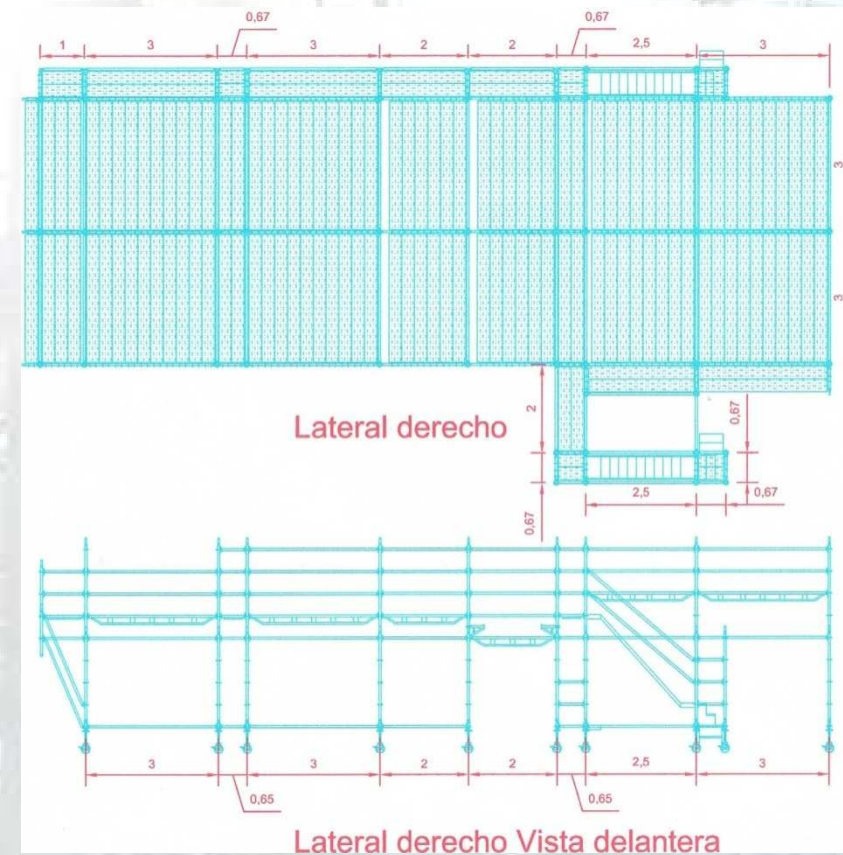
Planta y alzado de gradas para reparación de aviones
