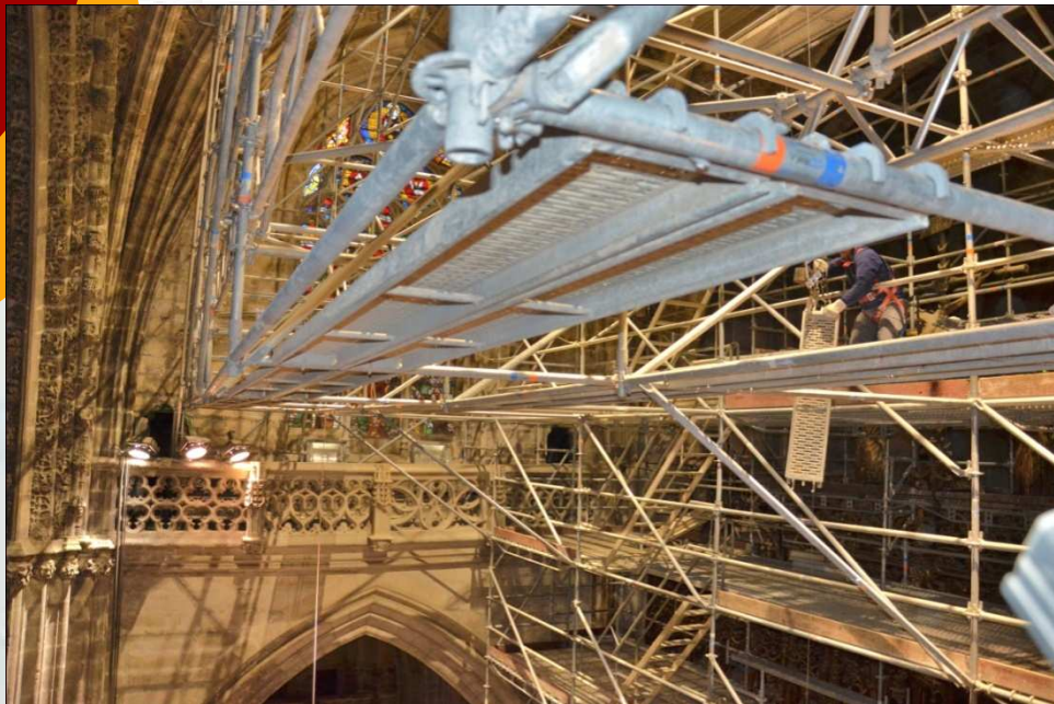
Bóveda del Presbiterio de la Catedral de Sevilla (Andamio volado sobre vigas de celosía de 15m de largo)
