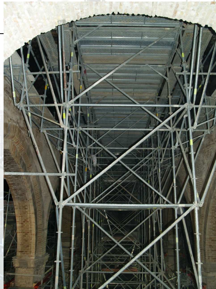
Apuntalamiento artesonado de la iglesia de Santa Catalina (Sevilla)
