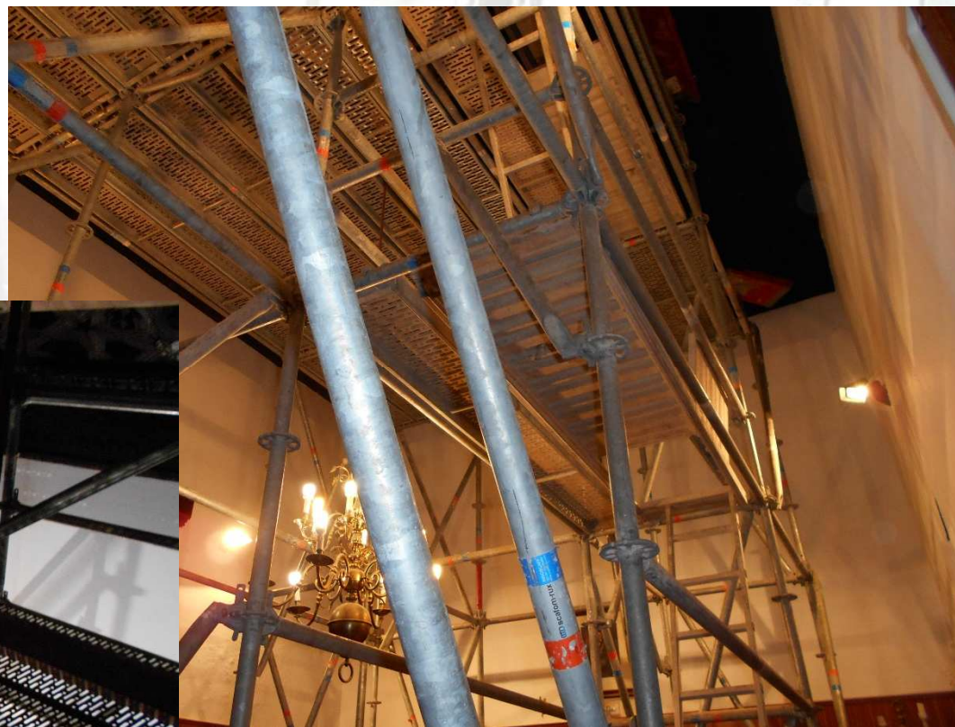
Sala de Audiencias, Juzgado de Marchena. Apuntalamiento de artesanado
