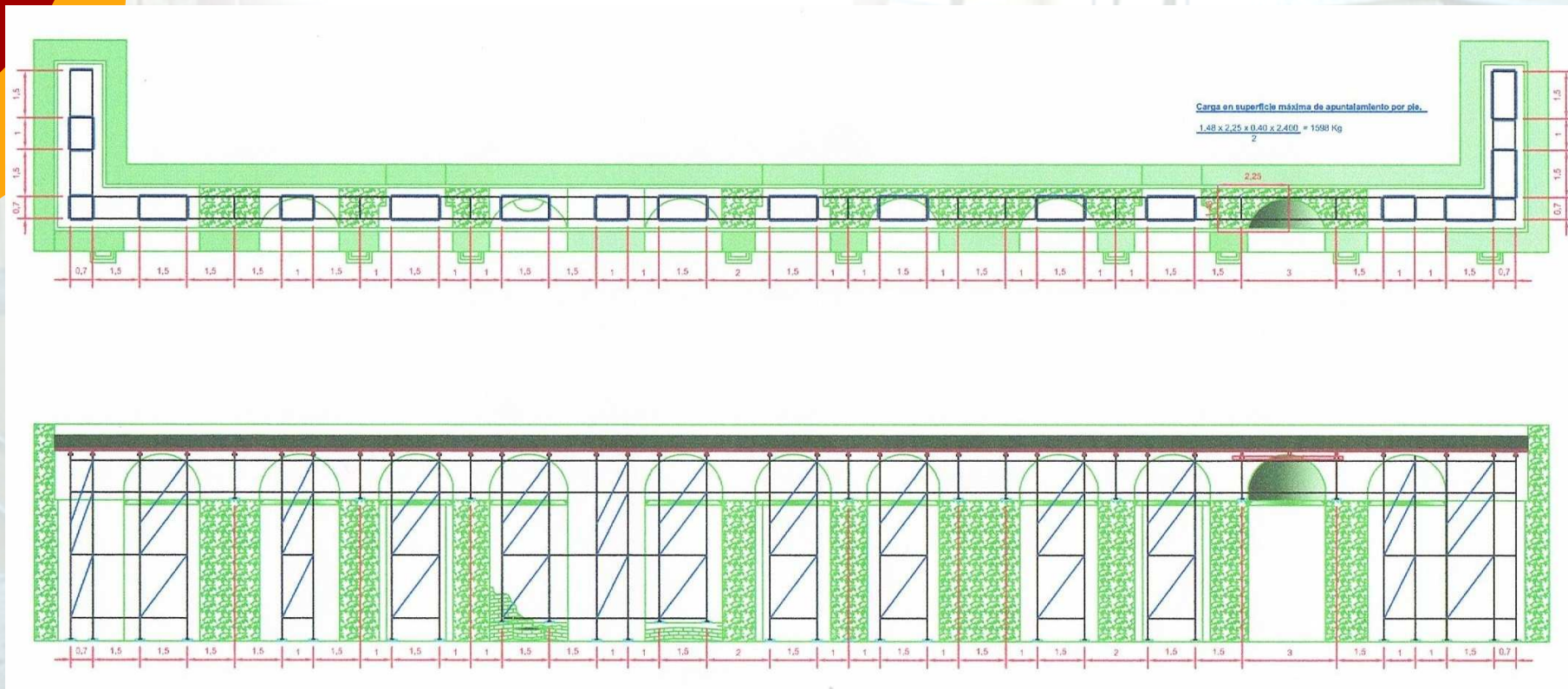
Planta y alzado apuntalamiento Teatro Romano de Itálica
