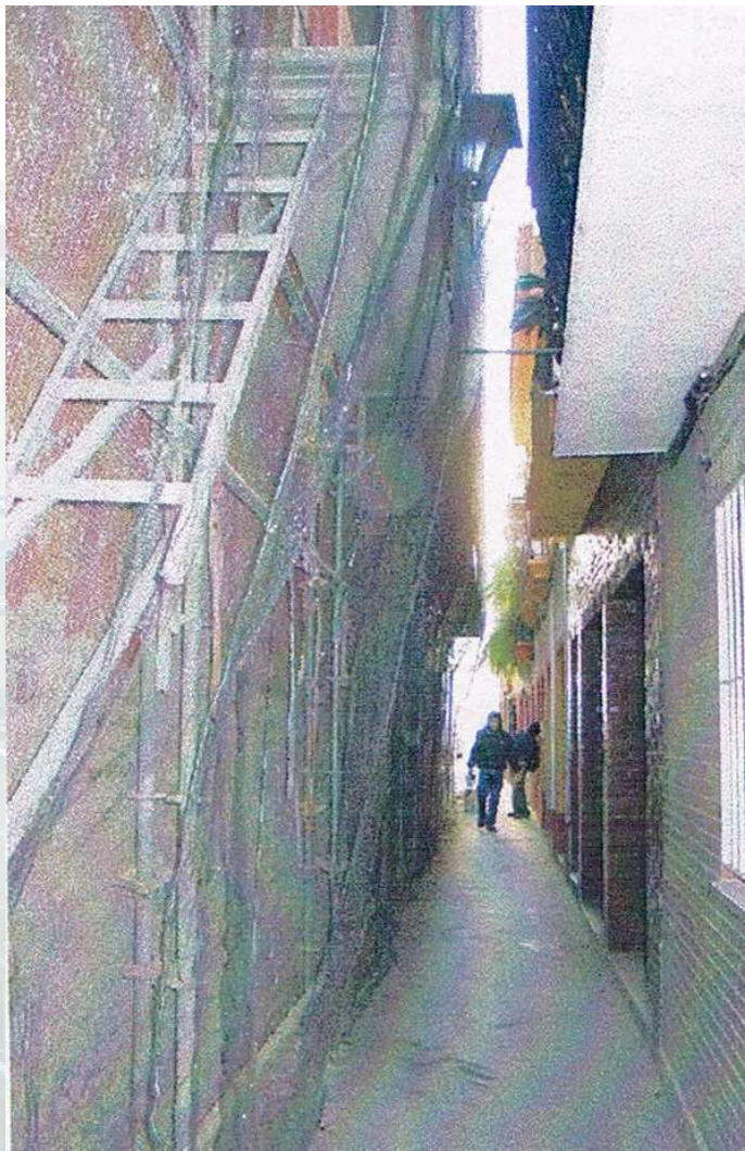
Andamio en calle peatonal muy estrecha. El sistema permite el transito de peatones.
