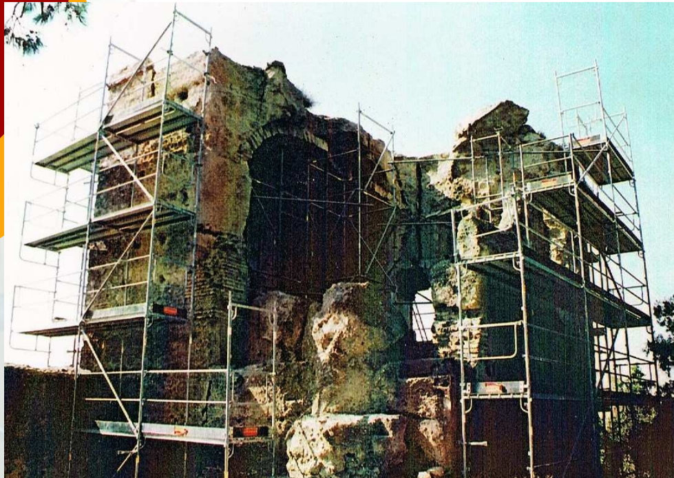
Castillo Luna Mairena del Alcor. Andamio exterior y apuntalamiento interior de bóvedas.
