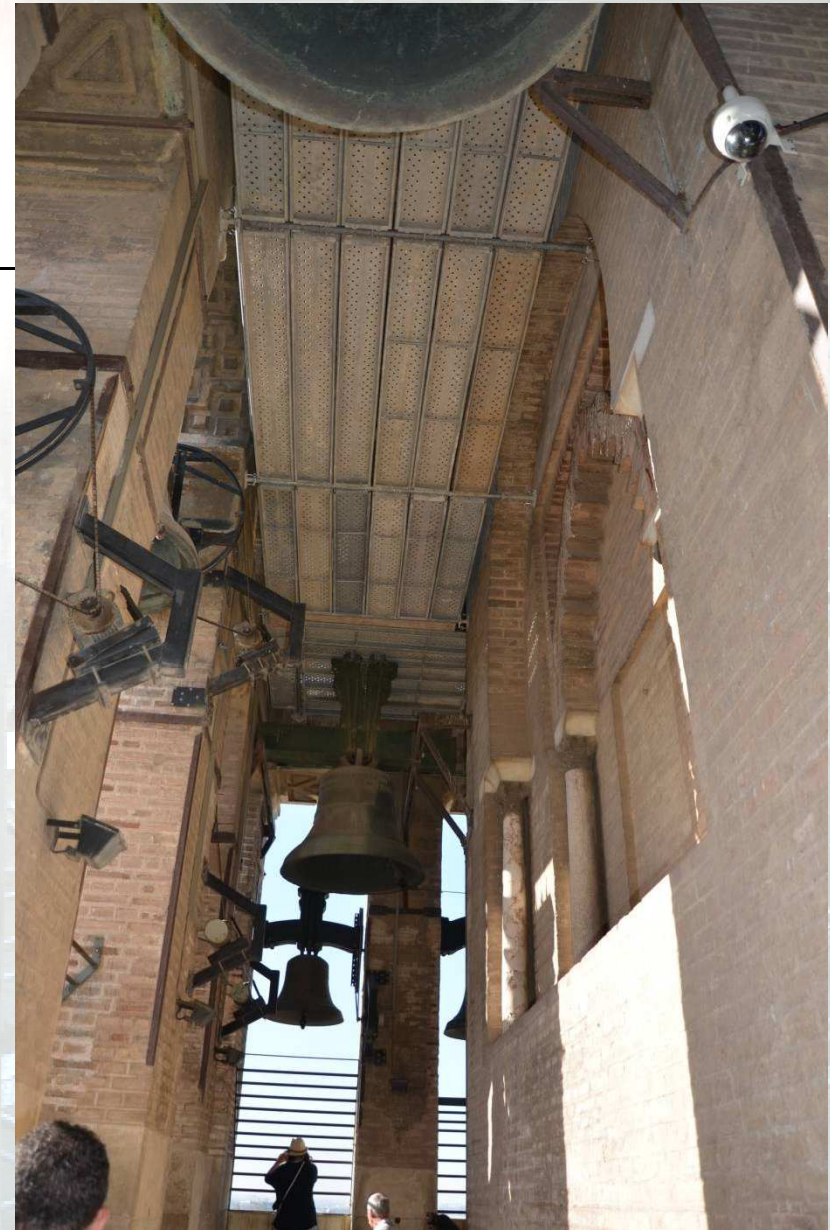
Plataforma para limpieza de las bóvedas del cuerpo de campanas de la Giralda. Como requerimiento no interferir al turismo.
